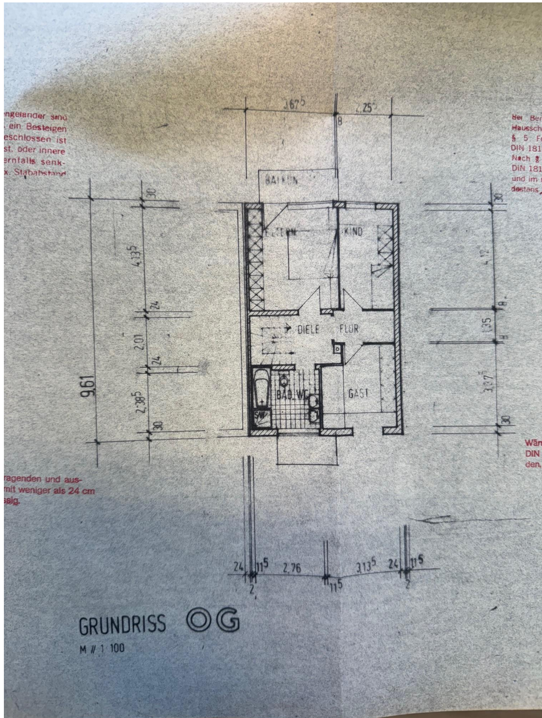
Grundriss Obergeschoss
