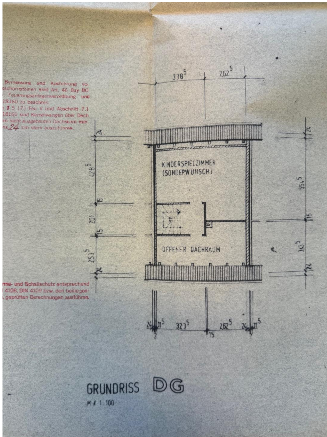
Grundriss Dachgeschoss
